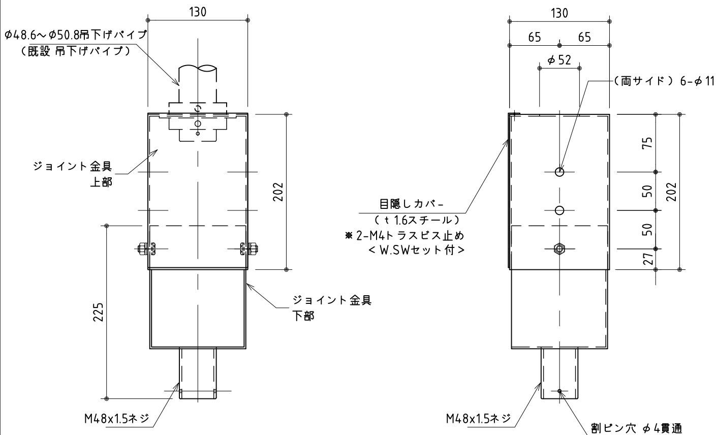
a部 詳細図 S=1/5
