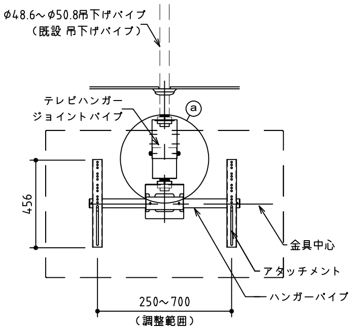
組込図 S=1/20
