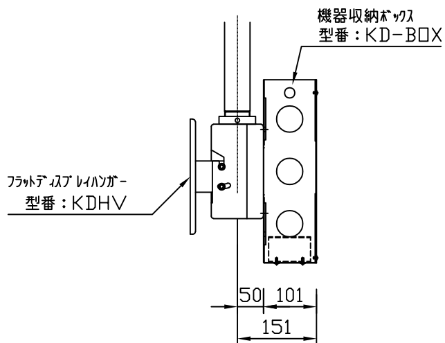
KD-BOX取付図
