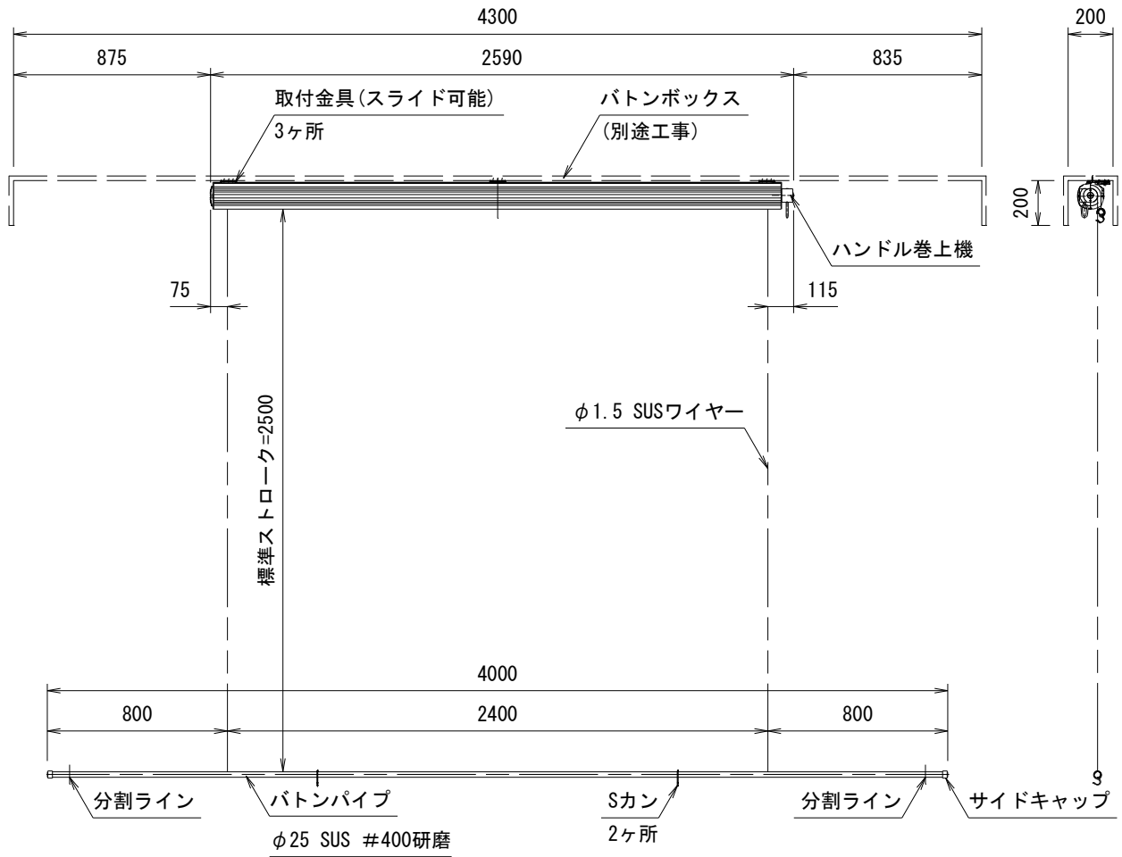
外観図 S=1/30
