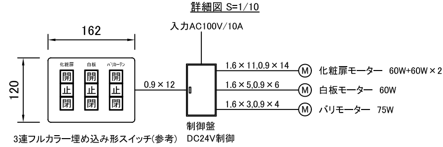
配線ブロック図
