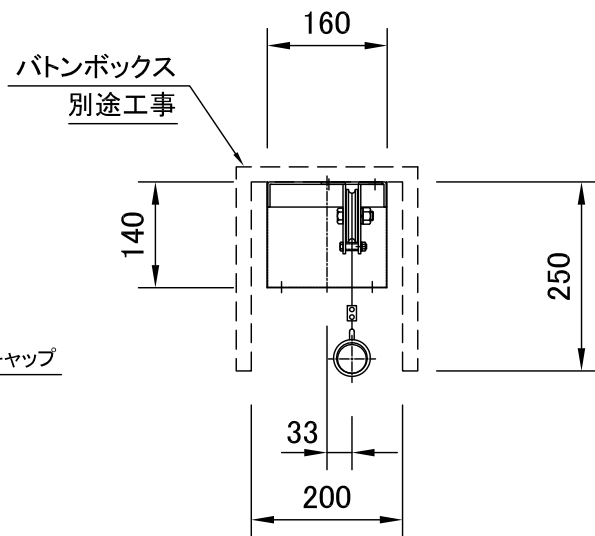
詳細図 S=1/10
