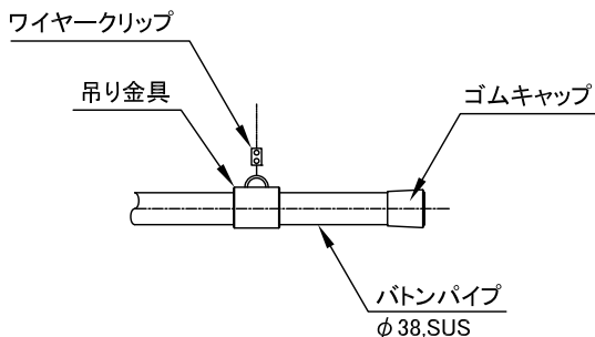
ボタンパイプ詳細図 S=1/10
