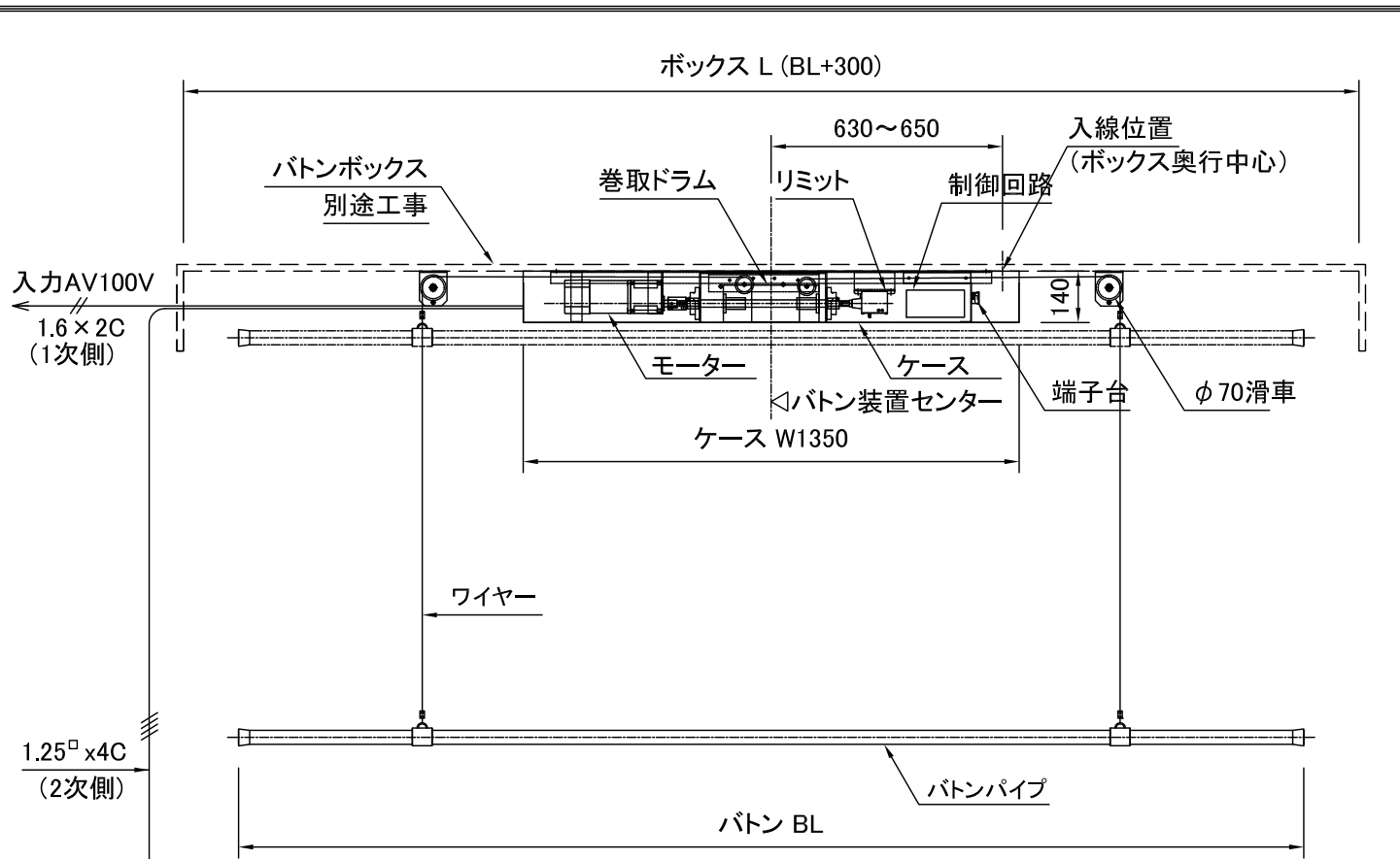
外観図 S=1/20
