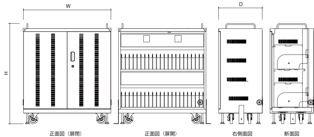
正面図 (扉閉)
