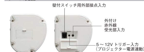
壁付スイッチ用外部接点入力 外付け赤外線受光部入力 5~12Vトリガー入力 (プロジェクター電源連動)
